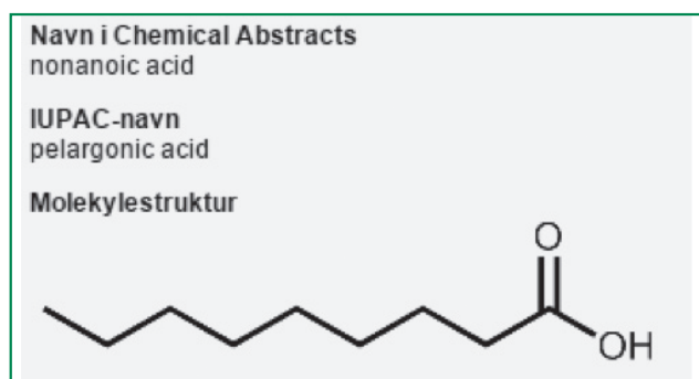
Figur 1: Pelargonsyre molekylestruktur.
